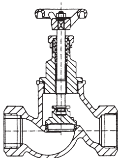
Fig. 1 - Valvola di intercettazione GXMZ
