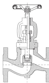
Fig. 2 - Valvola di intercettazione GXM16Z
