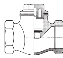
Fig. 5 - Valvola di ritegno RJ205N
