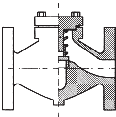
Fig. 3 - Valvola di ritegno RJ216Z
