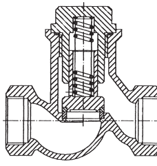
Fig. 4 - Valvola di ritegno RJ205Z
